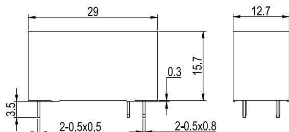
1A2 外形尺寸图
