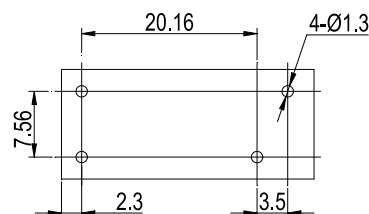
安装尺寸图 (底视图)
