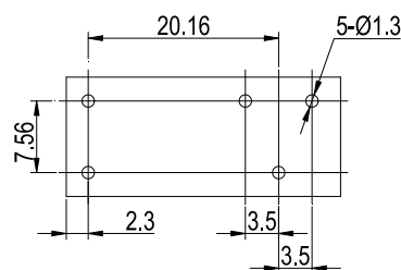
安装尺寸图 (底视图)
