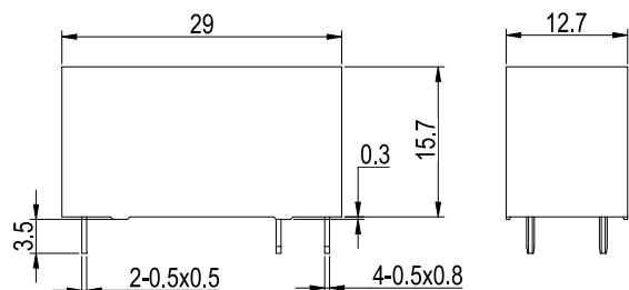
1C1 外形尺寸图
