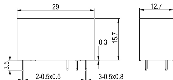
1C2 外形尺寸图
