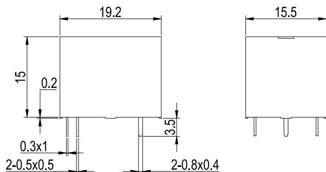
外形尺寸图
