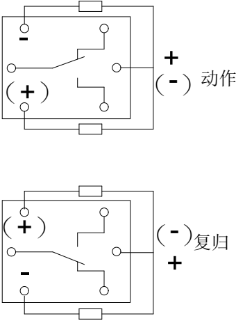
(底视图)
