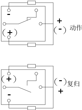
(底视图)
