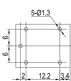
(底视图)
